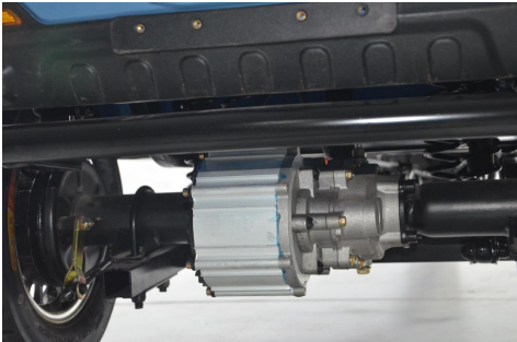
Motor
