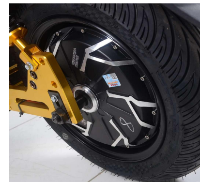
高速电机
